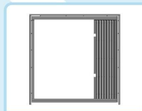
modelo14 Corredera derecha, no abatible, no levanta guía
