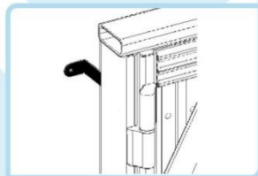
3.5 Orejetas desplazadas y solapadas
